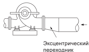
Рис. 26 Правильно смонтированный переходник
