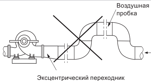
Рис. 32 Неправильно смонтированный всасывающий трубопровод
