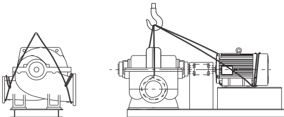
Рис. 15 Подъём насоса с низковольтным электродвигателем
