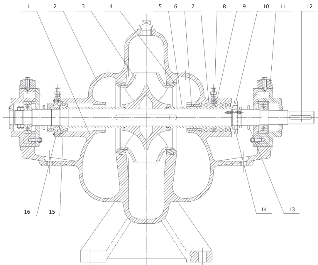
Рис. 42 Вид в разрезе, стандартный тип исполнения 2
