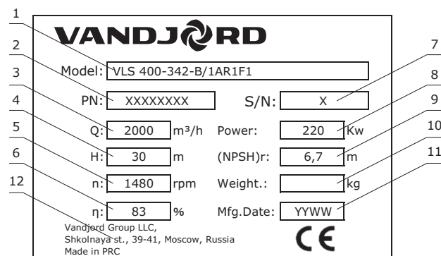
Рис. 13 Фирменная табличка насоса VLS
