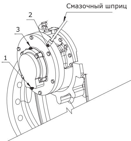
Рис. 38 Конструкция подшипника с консистентной смазкой
