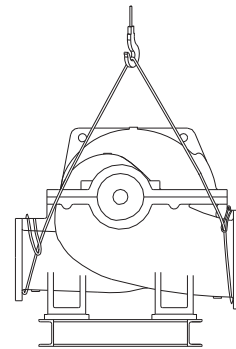
Рис. 17 Подъём одного насоса с опорной плитой
