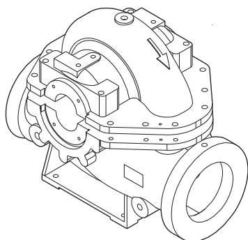
Рис. 6 Верхняя и нижняя части корпуса насоса VLS
