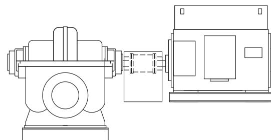
Рис. 5 Насос с электродвигателем и отдельными рамами-основаниями
