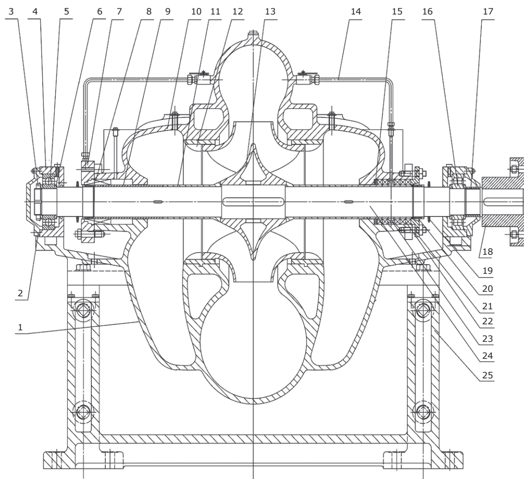
Рис. 43 Вид в разрезе, стандартный тип исполнения 3
