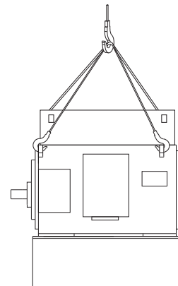
Рис. 19 Подъём высоковольтного электродвигателя с опорной плитой
