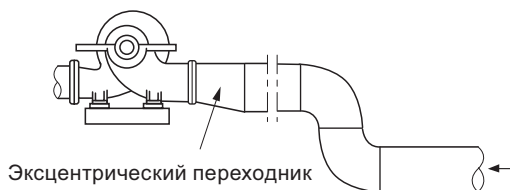
Рис. 31 Правильно смонтированный всасывающий трубопровод
