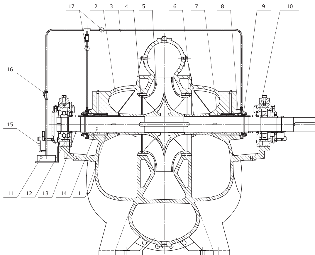
Рис. 46 Вид в разрезе, стандартный тип исполнения 6
