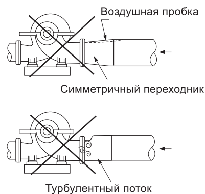
Рис. 27 Переходники, из-за которых образуются воздушные пробки и турбулентность
