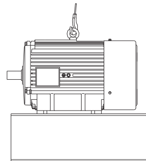
Рис. 18 Подъём низковольтного электродвигателя с опорной плитой
