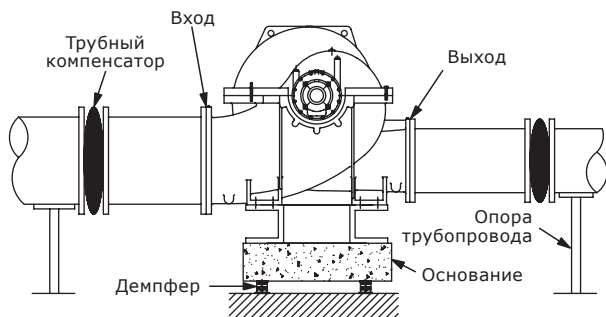
Рис. 24 Основание с демпфером и трубным компенсатором
