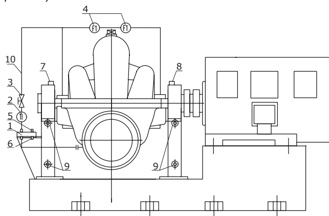
Рис. 20 Пример насоса в исполнении с системой охлаждения для перекачиваемых жидкостей с температурой выше 80 °С
