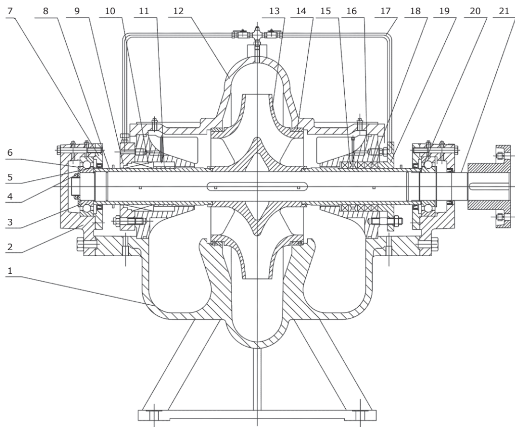
Рис. 41 Вид в разрезе, стандартный тип исполнения 1
