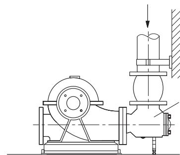
Рис. 35 Диффузор (1) во всасывающем трубопроводе
