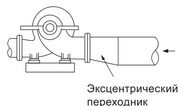
Рис. 28 Правильно смонтированный всасывающий трубопровод
