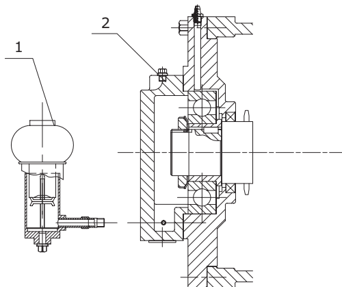
Рис. 39 Конструкция подшипника с масляной смазкой
