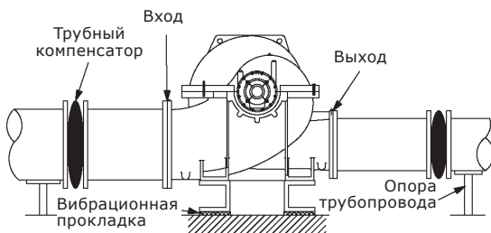
Рис. 25 Насос с вибрационной прокладкой
