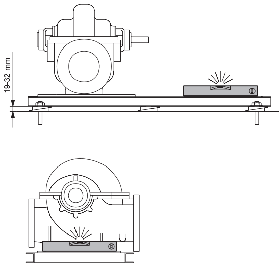
Рис. 22 Регулировка плиты-основания при помощи прокладок и выравнивание насоса
