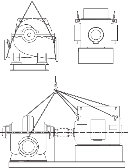
Рис. 16 Подъём насоса с высоковольтным электродвигателем
