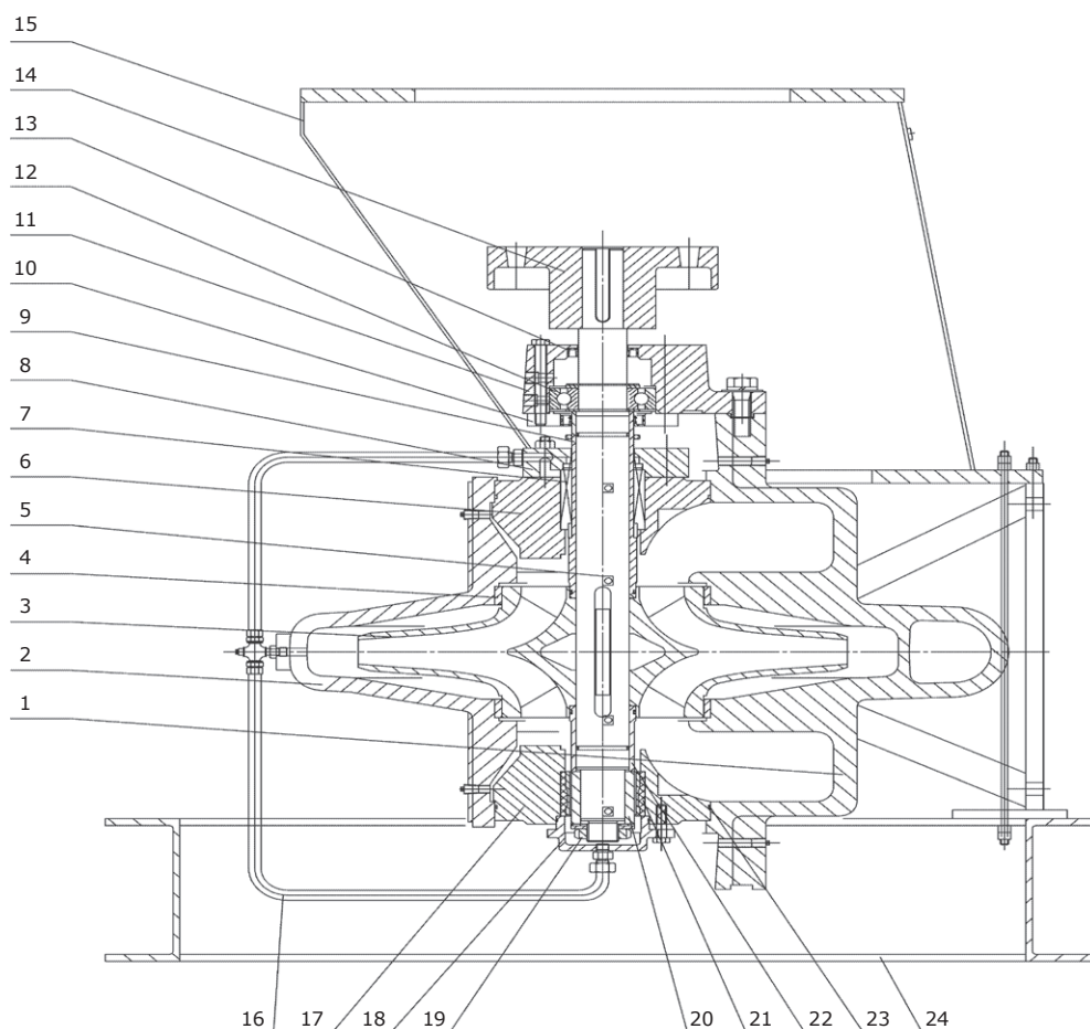
Рис. 44 Вид в разрезе, стандартный тип исполнения 4
