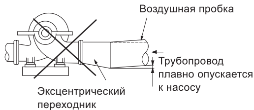
Рис. 30 Не правильно смонтированный всасывающий трубопровод
