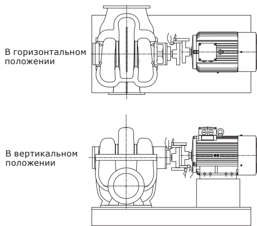
Рис. 37 Проверка соосности
