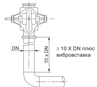
Рис. 33 Рекомендованный монтаж всасывающего трубопровода и длина прямого трубопровода между горизонтальным коленом и насосом
